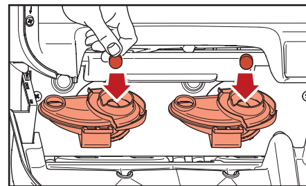
Fig. 5.4 - Insérez les pastilles de nettoyage Rinza.
