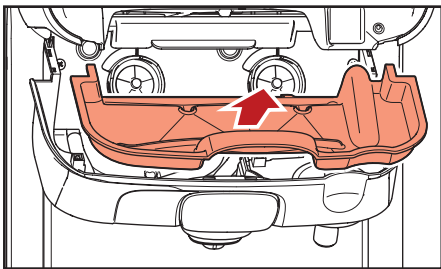
Fig. 5.11- Retirez le bac de récupération interne.
